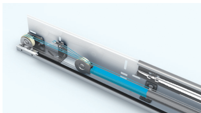
Système double ressorts et double câbles de levage
