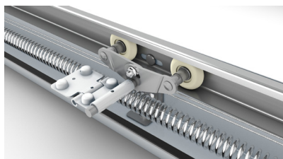
Double galets nylon sur roulement à bille
